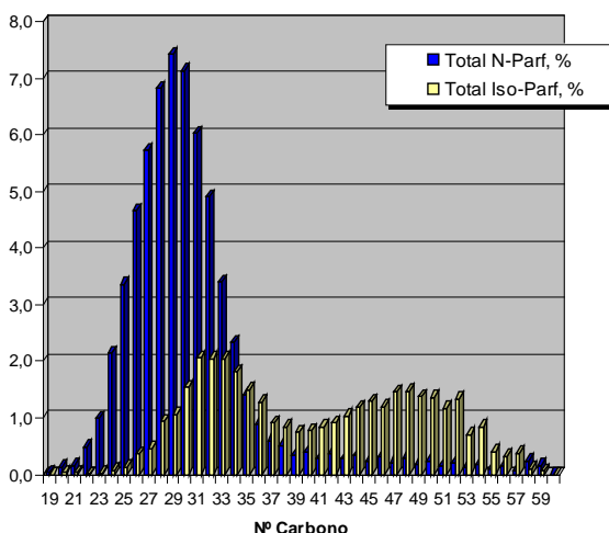
Distribución hidrocarbonada
